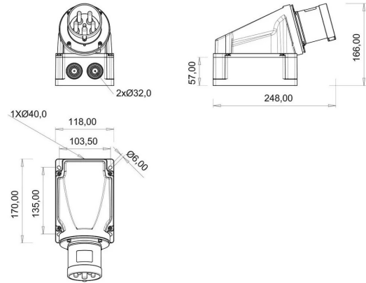
MASSZEICHNUNG
