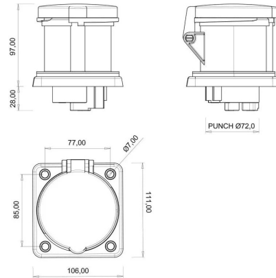
MASSZEICHNUNG
