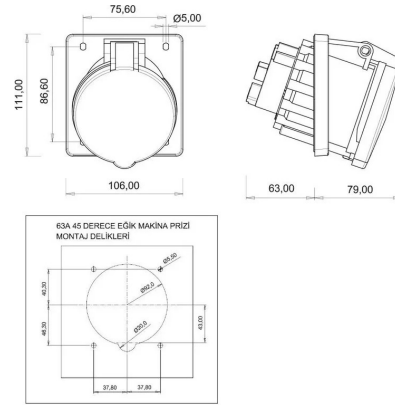
MASSZEICHNUNG
