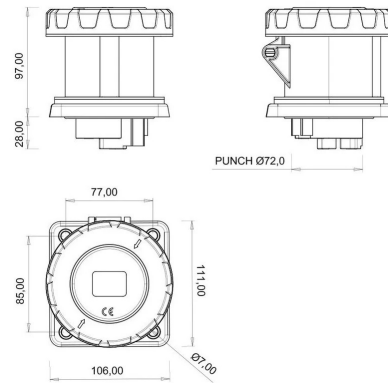
MASSZEICHNUNG
