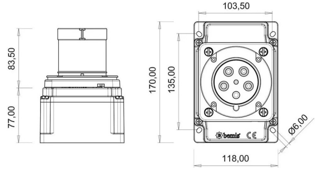
MASSZEICHNUNG
