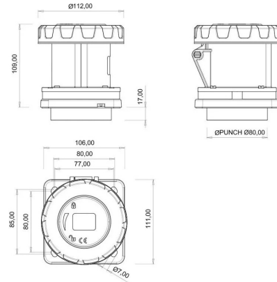
MASSZEICHNUNG
