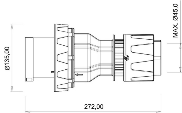
MASSZEICHNUNG
