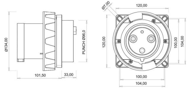
MASSZEICHNUNG
