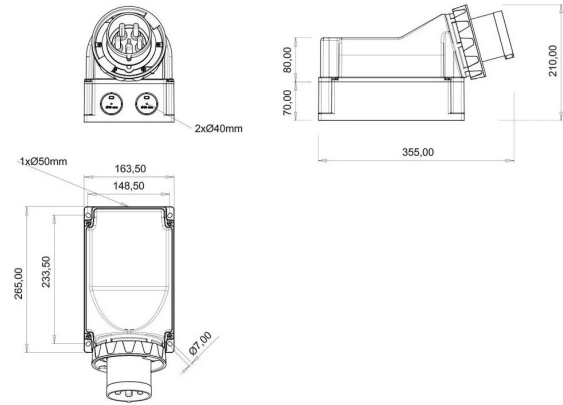
MASSZEICHNUNG
