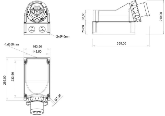
MASSZEICHNUNG
