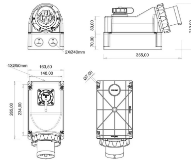
MASSZEICHNUNG
