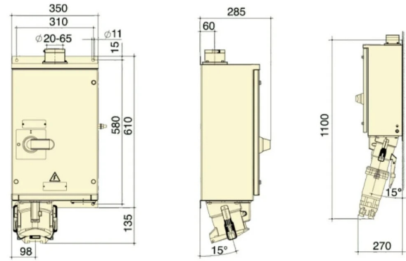
MASSZEICHNUNG
