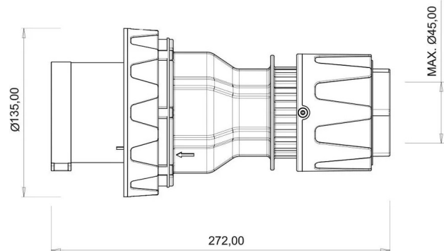
MASSZEICHNUNG
