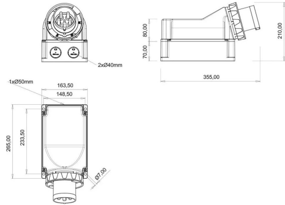
MASSZEICHNUNG
