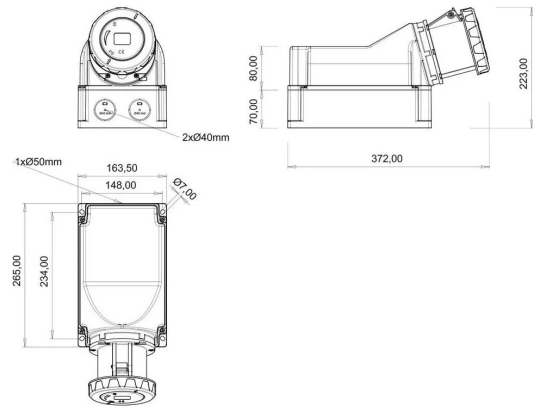
MASSZEICHNUNG
