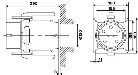
MASSZEICHNUNG
