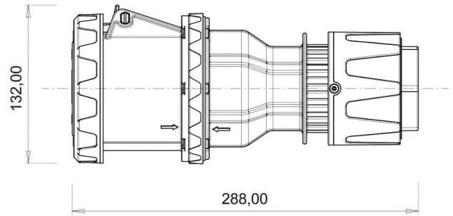
MASSZEICHNUNG
