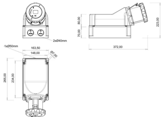
MASSZEICHNUNG
