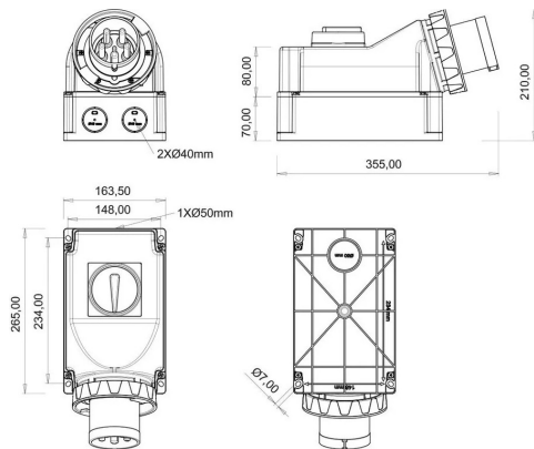
MASSZEICHNUNG
