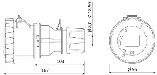
MASSZEICHNUNG
