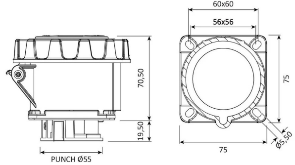
MASSZEICHNUNG
