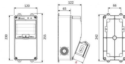
MASSZEICHNUNG
