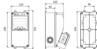
MASSZEICHNUNG
