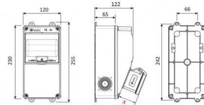
MASSZEICHNUNG
