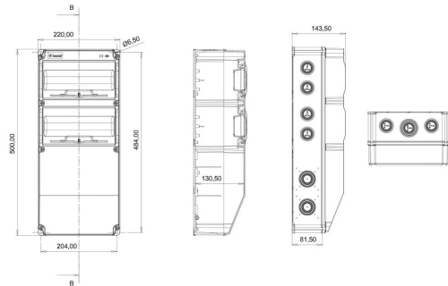
MASSZEICHNUNG
