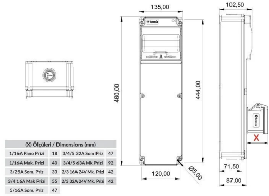
MASSZEICHNUNG
