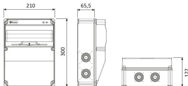
MASSZEICHNUNG
