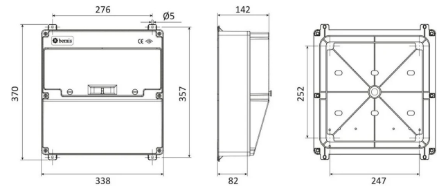
MASSZEICHNUNG
