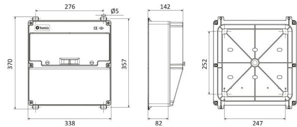
MASSZEICHNUNG
