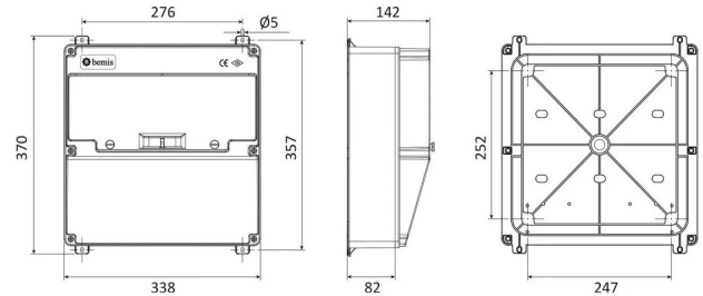
MASSZEICHNUNG
