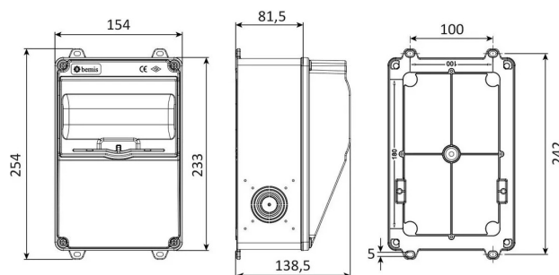
MASSZEICHNUNG
