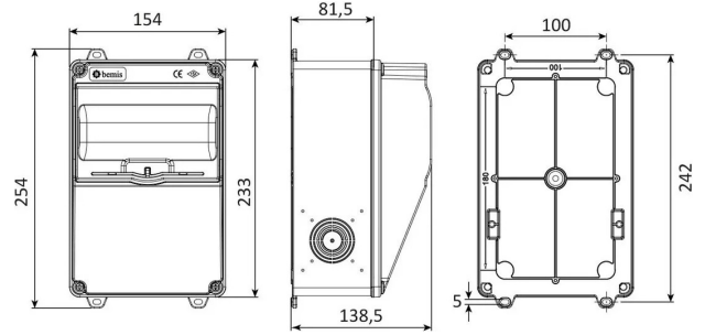
MASSZEICHNUNG
