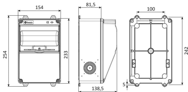
MASSZEICHNUNG
