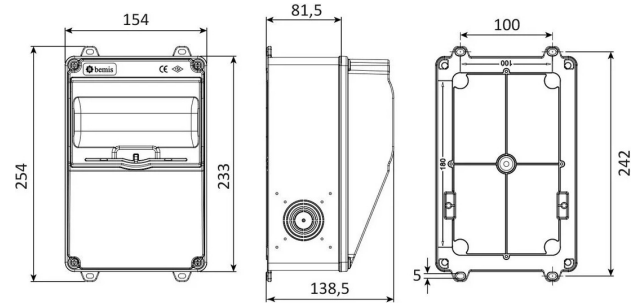
MASSZEICHNUNG
