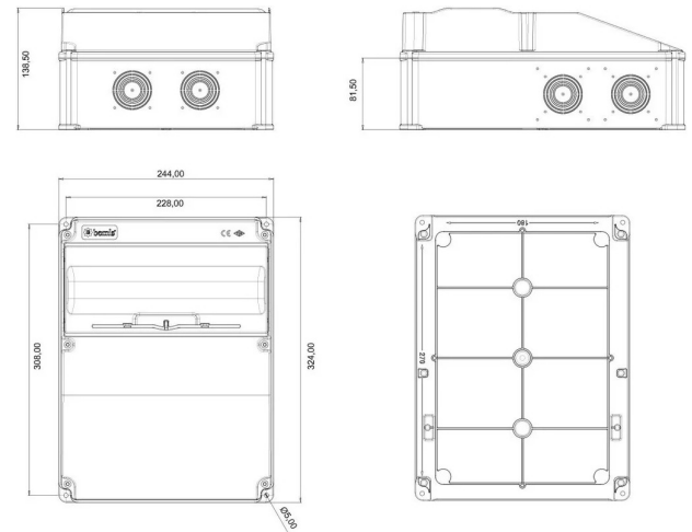
MASSZEICHNUNG
