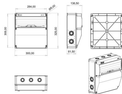
MASSZEICHNUNG
