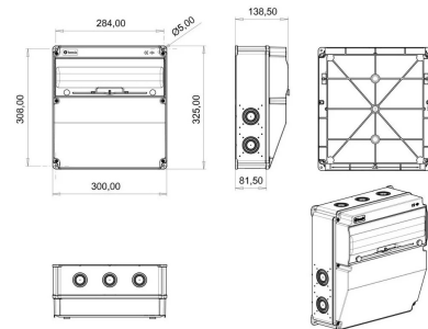
MASSZEICHNUNG
