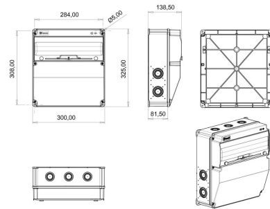
MASSZEICHNUNG
