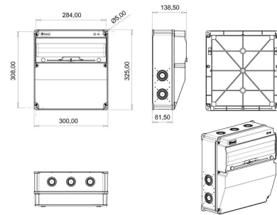
MASSZEICHNUNG
