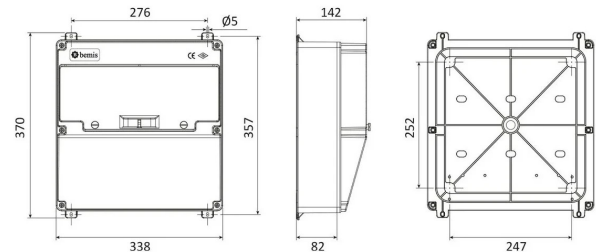
MASSZEICHNUNG
