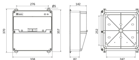
MASSZEICHNUNG
