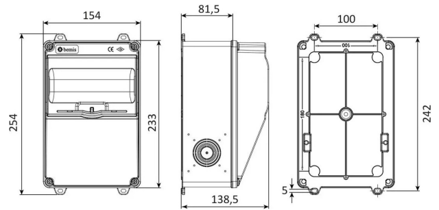
MASSZEICHNUNG
