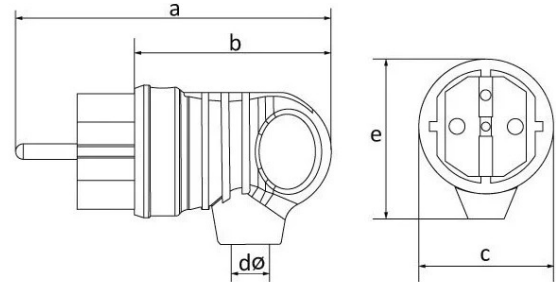
MASSZEICHNUNG
