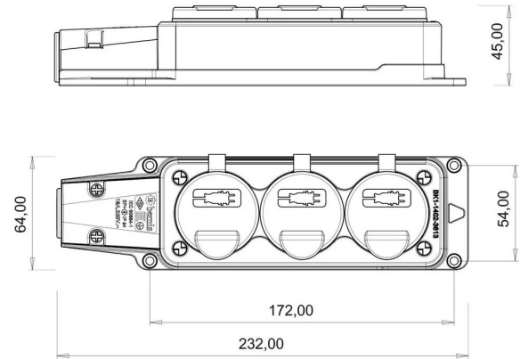
MASSZEICHNUNG
