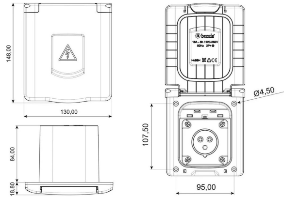
MASSZEICHNUNG
