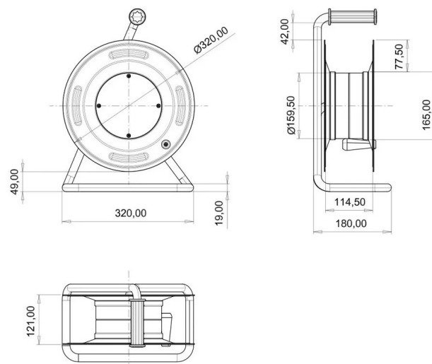
MASSZEICHNUNG
