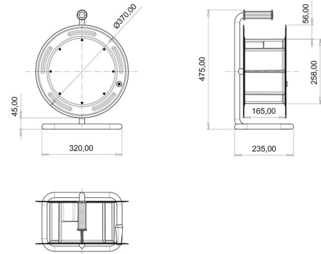
MASSZEICHNUNG
