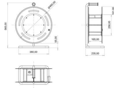
MASSZEICHNUNG
