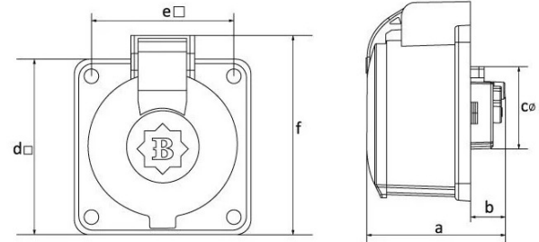
Ölçüler / Dimensions (mm)
