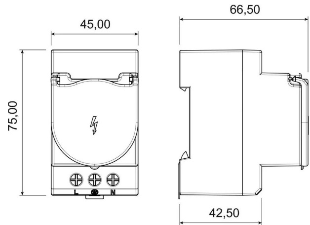
MASSZEICHNUNG
